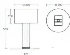
réf. 10505 ● 3 lampes standard perle 60 watts (E 27)
