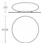
réf. 10511/1 ● 4 lampes sphériques perle 40 watts (E 27)
